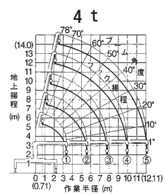
5段ブーム
