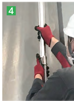
4 つっぱり棒のレバーロックを解除し伸縮部を天井まで伸ばす
