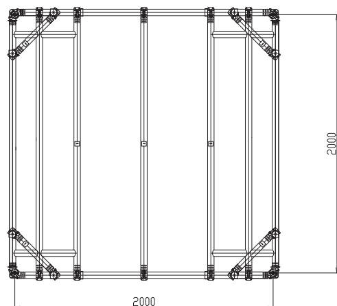
寸法図
