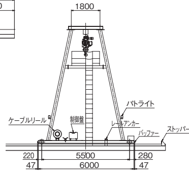
A-A矢視図
