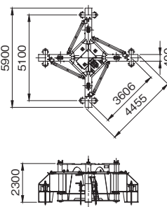
折畳架台仕様 (標準)
