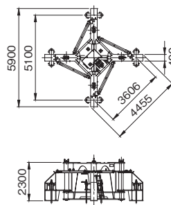
折畳架台仕様 (標準)
