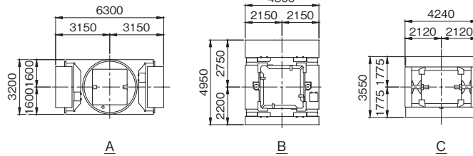
伸縮架台仕様 (オプション)
