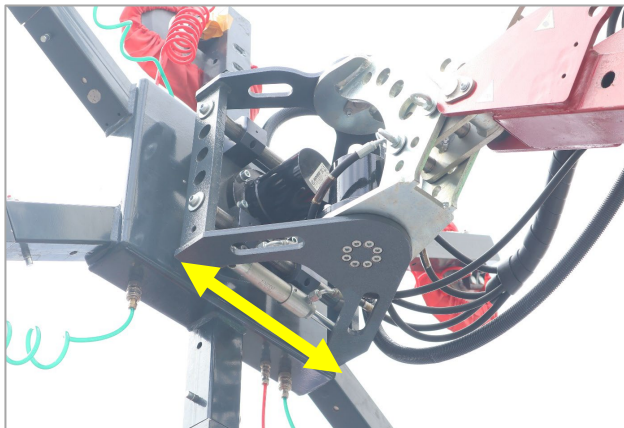
シリンダーが真横に水平移動し、微調整が可能
