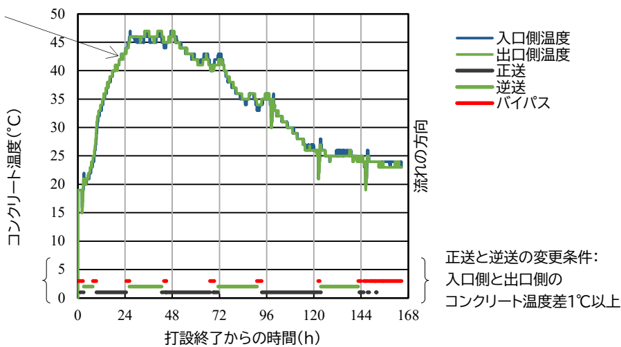
【図-4 コンクリート温度と流方向】
