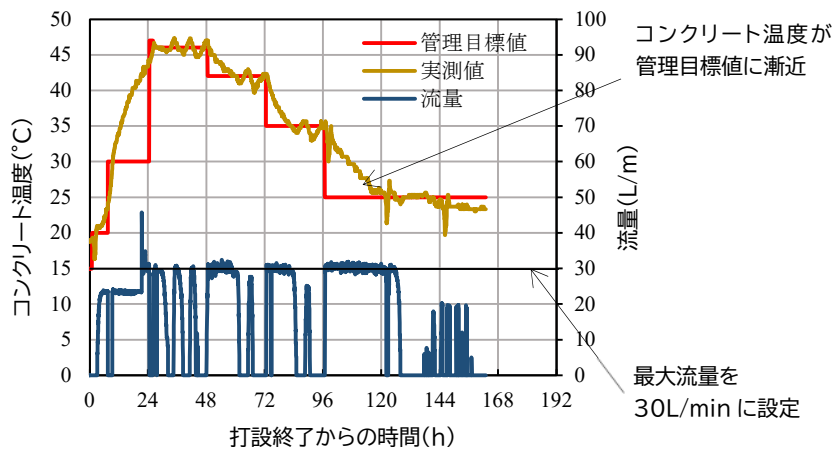
【図-3 コンクリート温度と流量】
