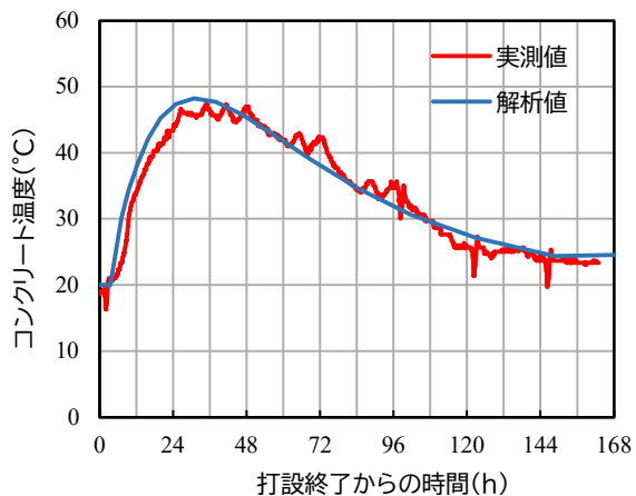
【図-5 解析と実験のコンクリート温度】
