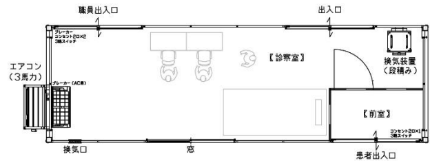
[B] 前室 1 室 (患者側のみ)
