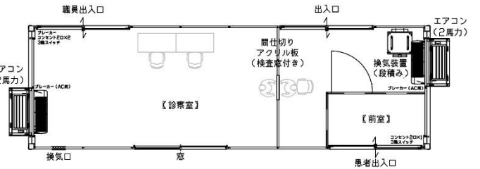
[E] 前室 1 室 (患者側のみ)、アクリル板で仕切りあり
