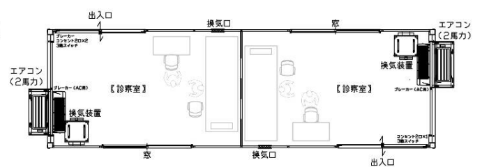
[H] 前室なし
