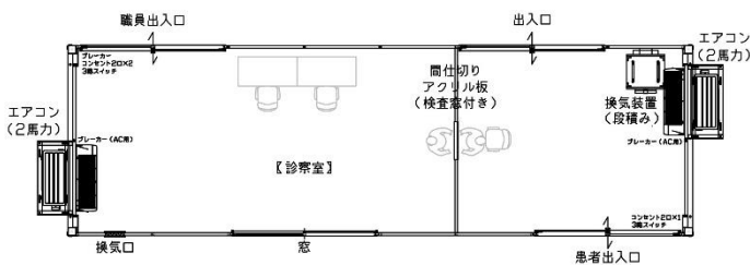
[F] 前室なし、アクリル板で仕切りあり
