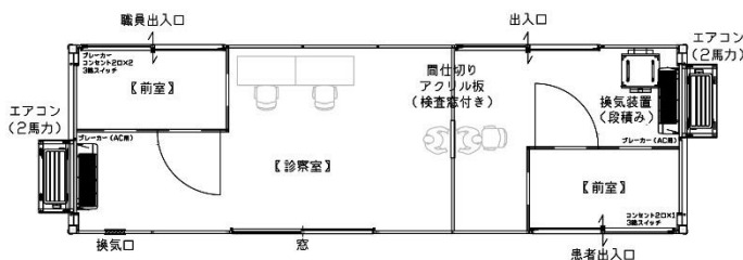
[D] 前室 2 室、アクリル板で仕切りあり
