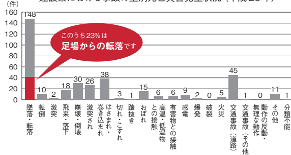
建設業における事故の型別死亡災害発生状況(平成26年)
