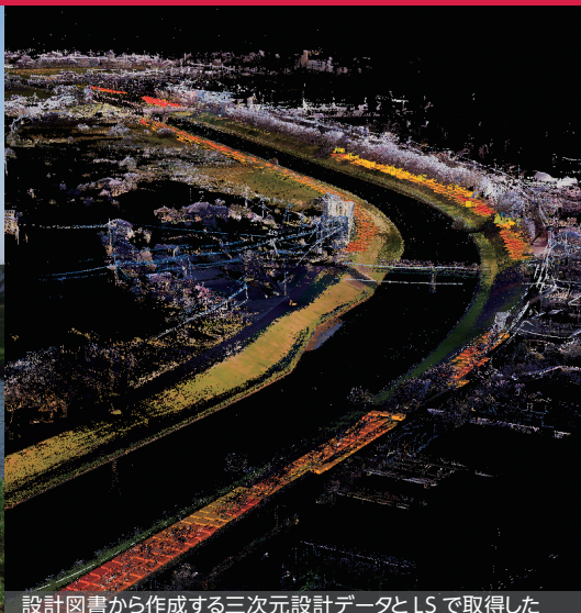
設計図書から作成する三次元設計データとLSで取得した三次元現況地形データの比較による土量算出
